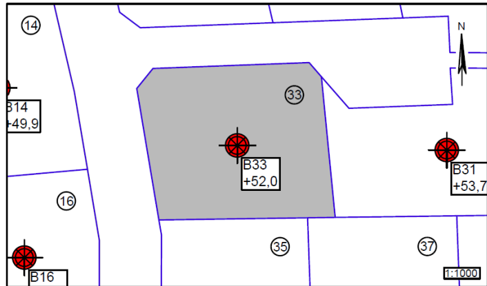
Figur 1 – Situationsplan 1:1000, Hus nr. 33
